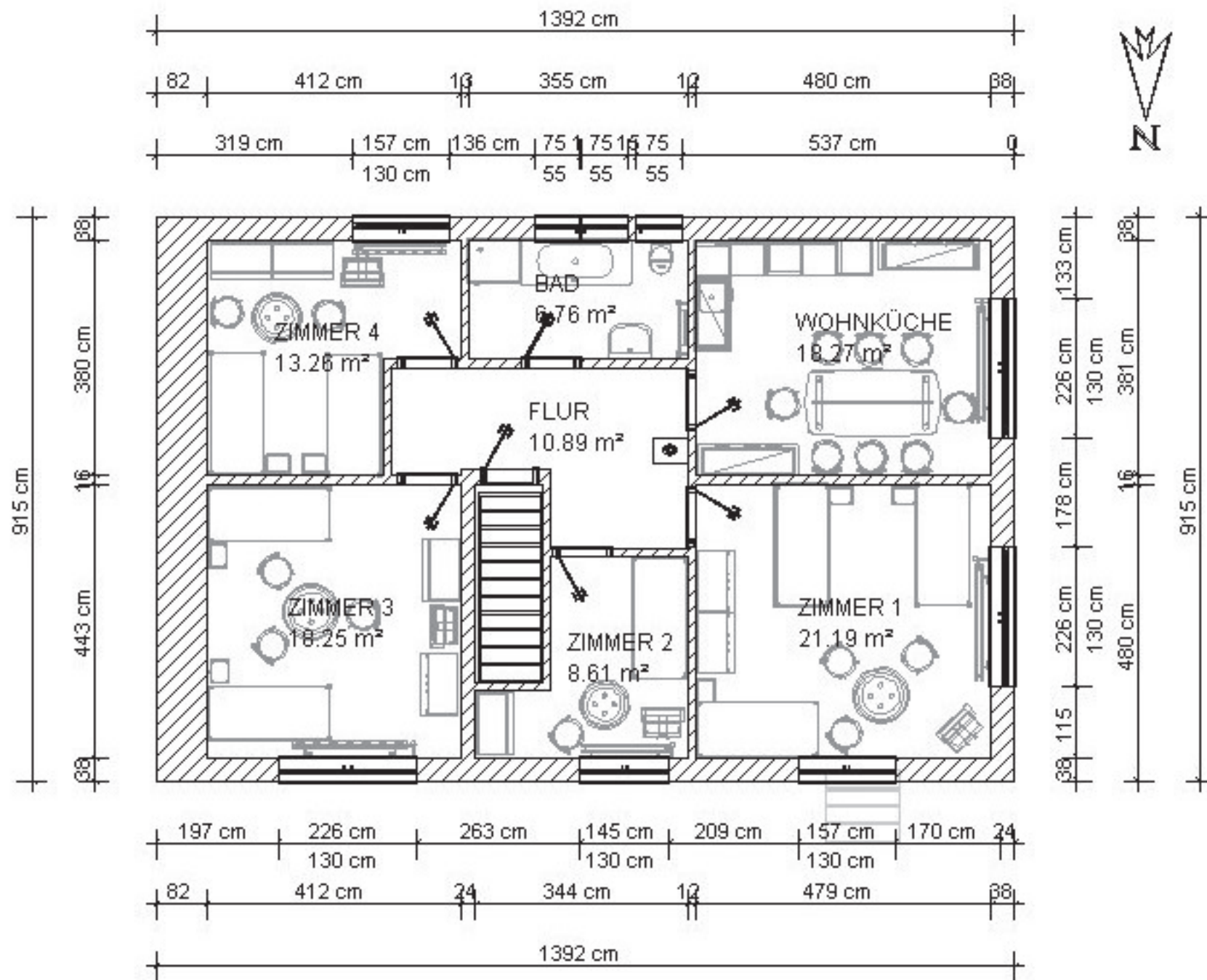
OBERGESCHOSS M 1:100 Wohnfläche ca.: 97,23 m 2
